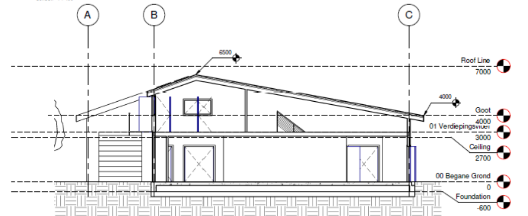
Referentie: A002 Doorsnede B-B schaal: 1 : 100
