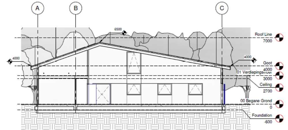
Referentie: A002 Doorsnede B-B schaal: 1 : 100
